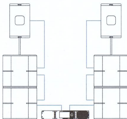
Système stéréo : 1 x P12 (passive) montée sur mât avec 2 x caissons L15 par côté
