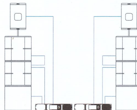
Système de façade moyen : (par côté) 1 x P12 (active) posée sur 2 x caissons L15 et 1 x caisson L15 (mode cardioïde)
