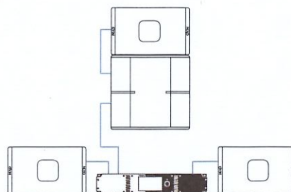
Système de retours : 1 x P12 horizontale sur 1 x caisson L15 (Drum Fill) + 2 x P12 horizontales en retours
